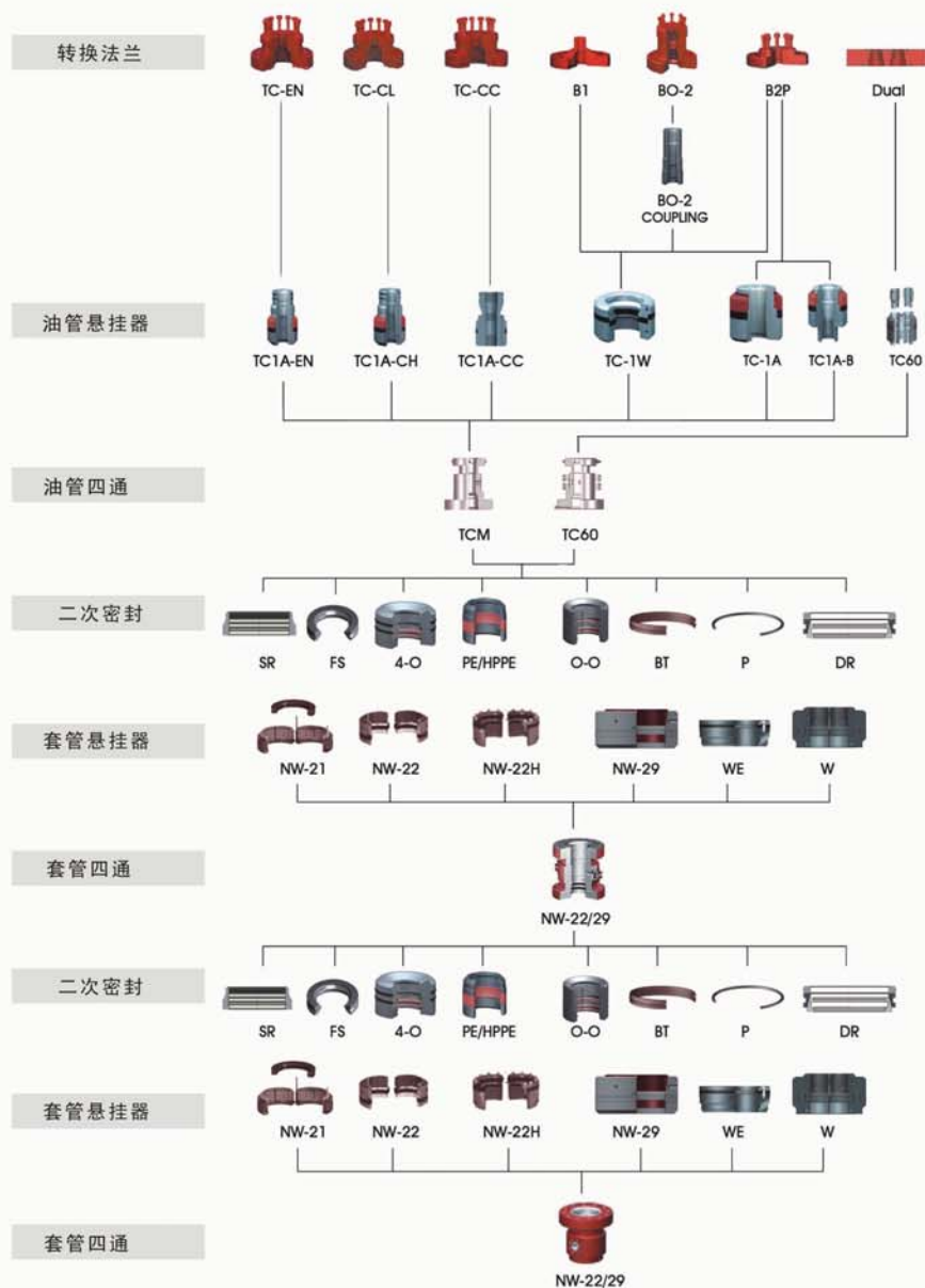
井口零件选择表
